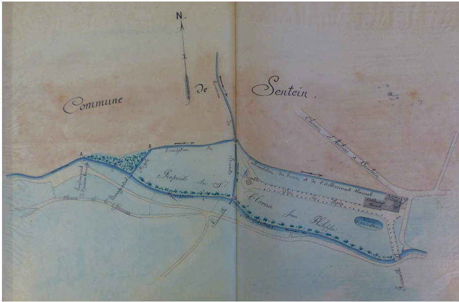
Fig. 9 : Plan de la station thermale de Sentein, 9 août 1897. AD Ariège, 7 S 693. © Archives départementales de l'Ariège.
