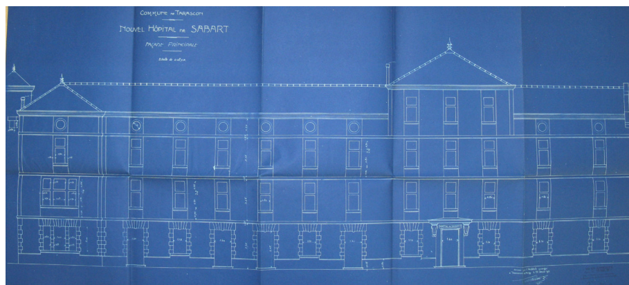
Élévation principale du projet de l'architecte Bacou, 18 janvier 1920. Archives départementales de l'Ariège, 1 X 105.
